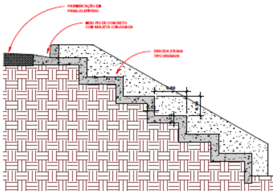
2 CORTE DESCIDA D'ÁGUA 1 : 25
