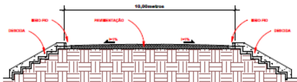
1 CORTE DA PAVIMENTAÇÃO 1 : 100
